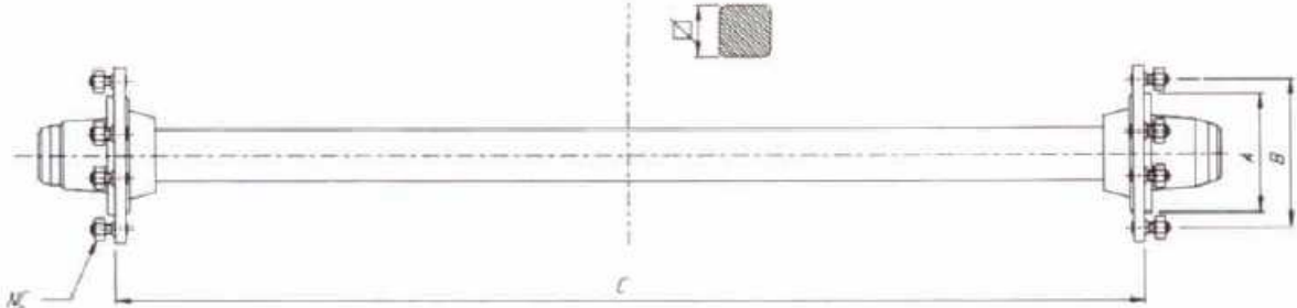
assale senza freno
